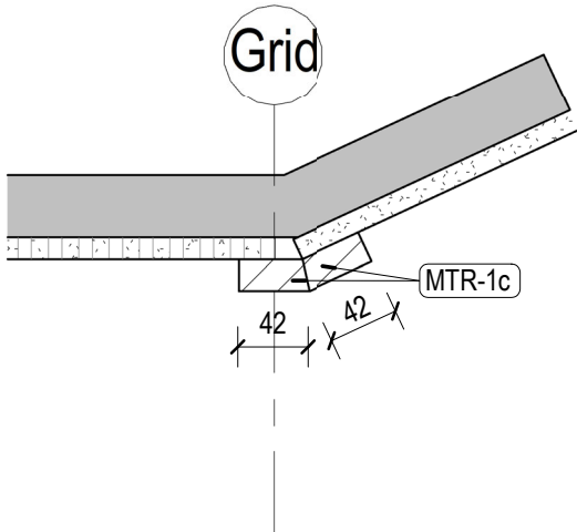
2 Raking Ceiling 1 : 5
